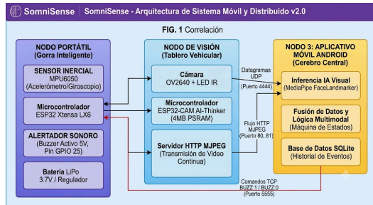
Fig. 1. Diagrama de bloques del sistema distribuido de alerta de fatiga: organización de los nodos portátiles y centrales, interfaces de comunicación inalámbrica y periféricos de salida física.
